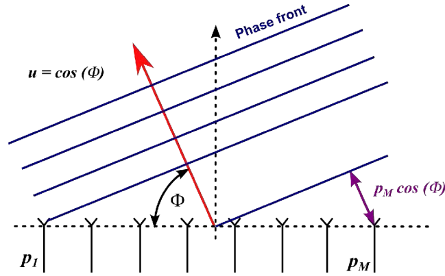
Figure 4: Linear antenna array
